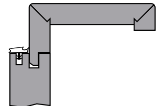
ZARGE MIT KLEINER RUNDKANTE, 100 MM BEKLEIDUNG FRAME WITH SMALL ROUNDED EDGE, 100 MM CASING
